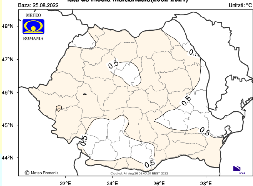
Abaterea temperaturii medii a aerului in perioada 05/09/2022 - 12/09/2022 fata de media multianuala(2002-2021)
