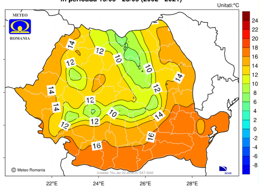
Media multianuala a temperaturii aerului la 2 m in perioada 19/09 - 26/09 (2002 - 2021)
