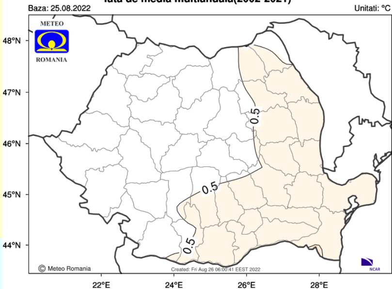
Abaterea temperaturii medii a aerului in perioada 19/09/2022 - 26/09/2022 fata de media multianuala(2002-2021)
