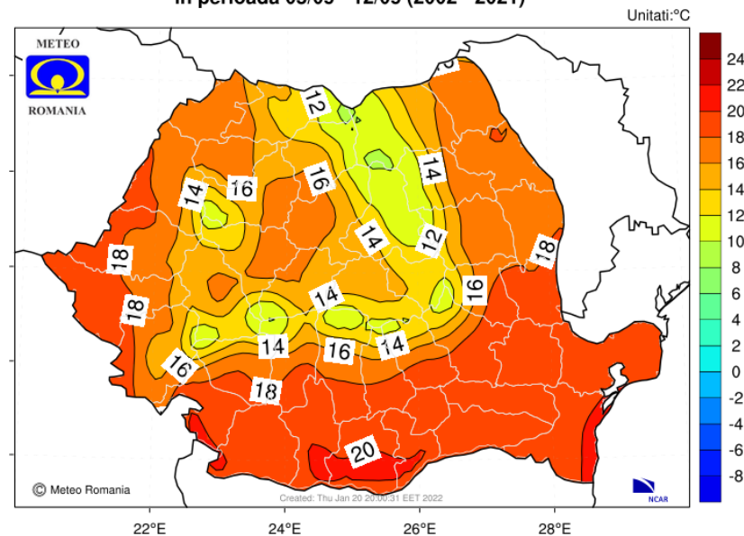
Media multianuala a temperaturii aerului la 2 m in perioada 05/09 - 12/09 (2002 - 2021)
