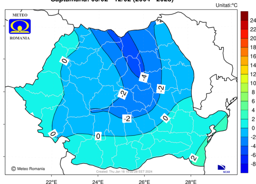
Media multianuala a temperaturii aerului la 2 m Saptamana: 05/02 - 12/02 (2004 - 2023)
