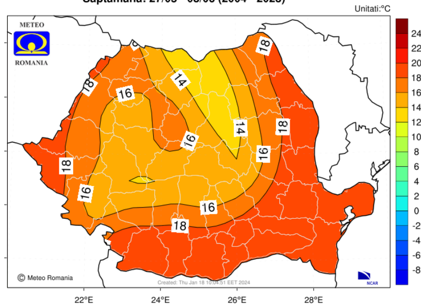
Media multianuala a temperaturii aerului la 2 m Saptamana: 27/05 - 03/06 (2004 - 2023)
