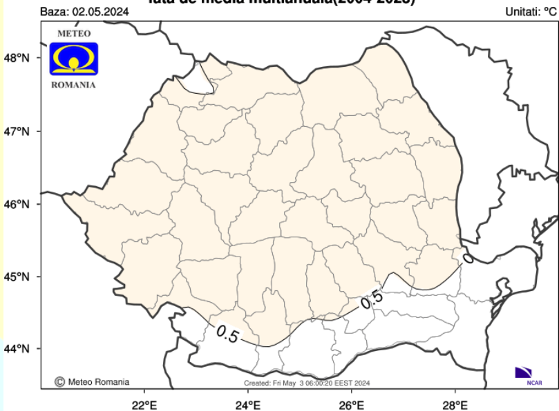
Abaterea temperaturii medii a aerului in perioada 27/05/2024 - 03/06/2024 fata de media multianuala(2004-2023)
