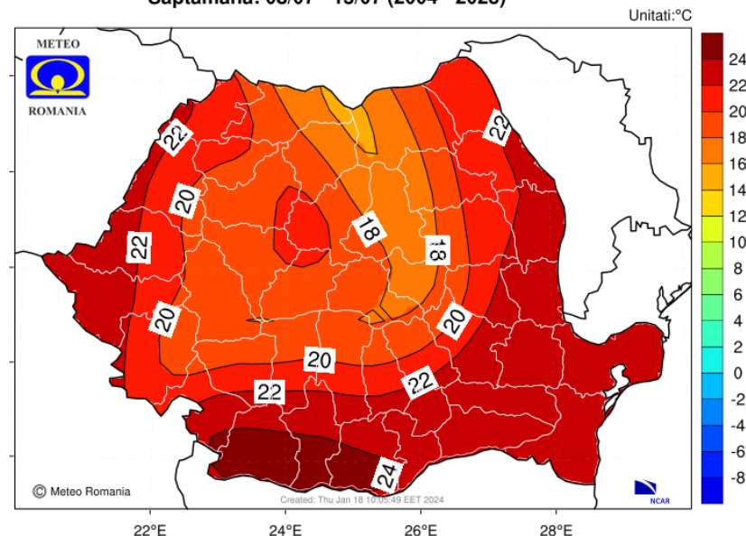
Media multianuala a temperaturii aerului la 2 m Saptamana: 08/07 - 15/07 (2004 - 2023)
