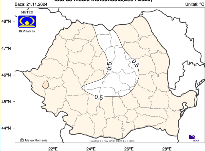
Abaterea temperaturii medii a aerului in perioada 16/12/2024 - 23/12/2024 fata de media multianuala(2004-2023)
