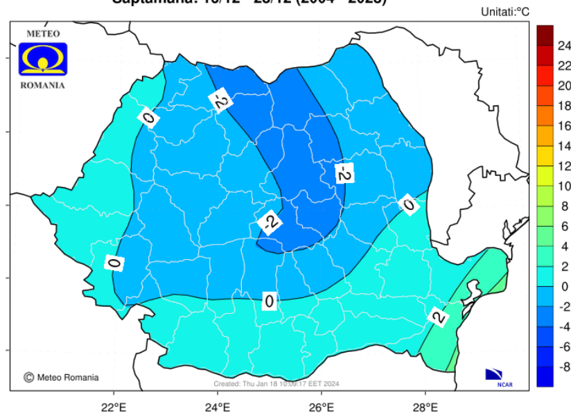
Media multianuala a temperaturii aerului la 2 m Saptamana: 16/12 - 23/12 (2004 - 2023)
