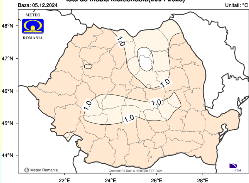
Abaterea temperaturii medii a aerului in perioada 23/12/2024 - 30/12/2024 fata de media multianuala(2004-2023)
