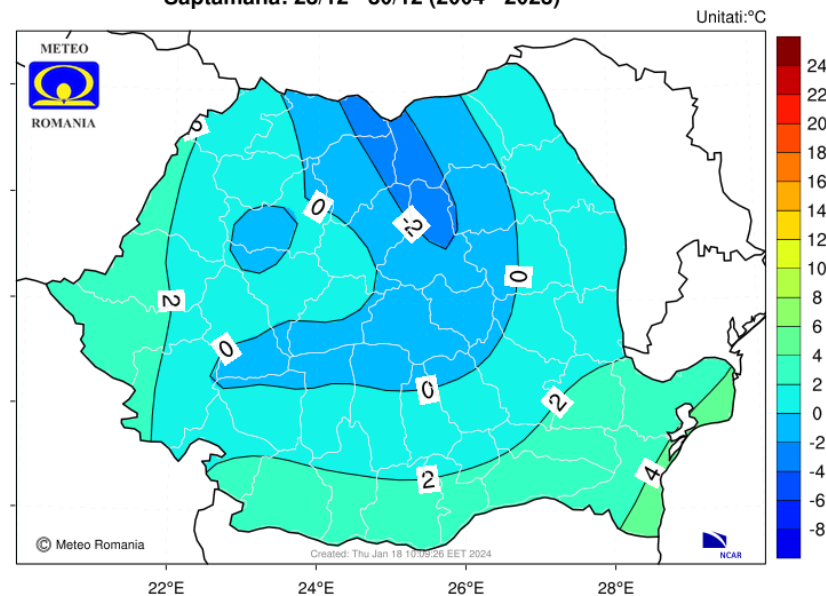
Media multianuala a temperaturii aerului la 2 m Saptamana: 23/12 - 30/12 (2004 - 2023)
