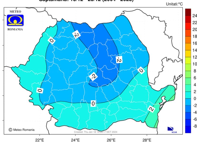
Media multianuala a temperaturii aerului la 2 m Saptamana: 16/12 - 23/12 (2004 - 2023)
